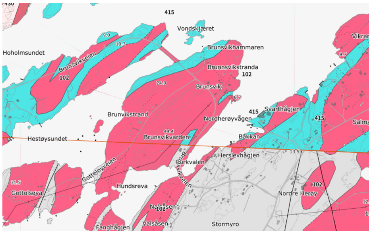
Figur 3: Planområdet består hovedsakelig av bergartene granitt og granodioritt (rød farge) og et område med marmor, vesentlig kalkspatmarmor (blå farge).
