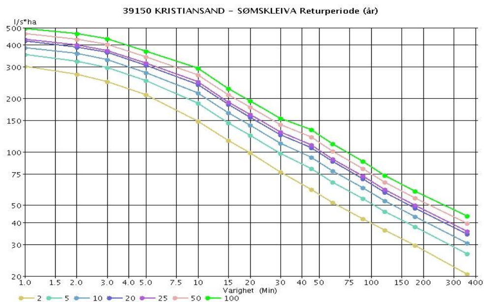
Figur 7 IVF-kurve fra stasjonen 39150 Kristiansand - Sømkleiva
