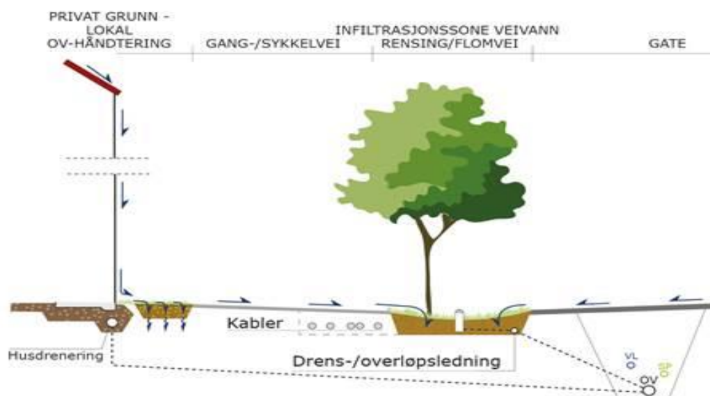
Figur 5 Lokal fordøyningsanlegg (© - COWI - Svein Ole Åstebøl/Simona Robba)
