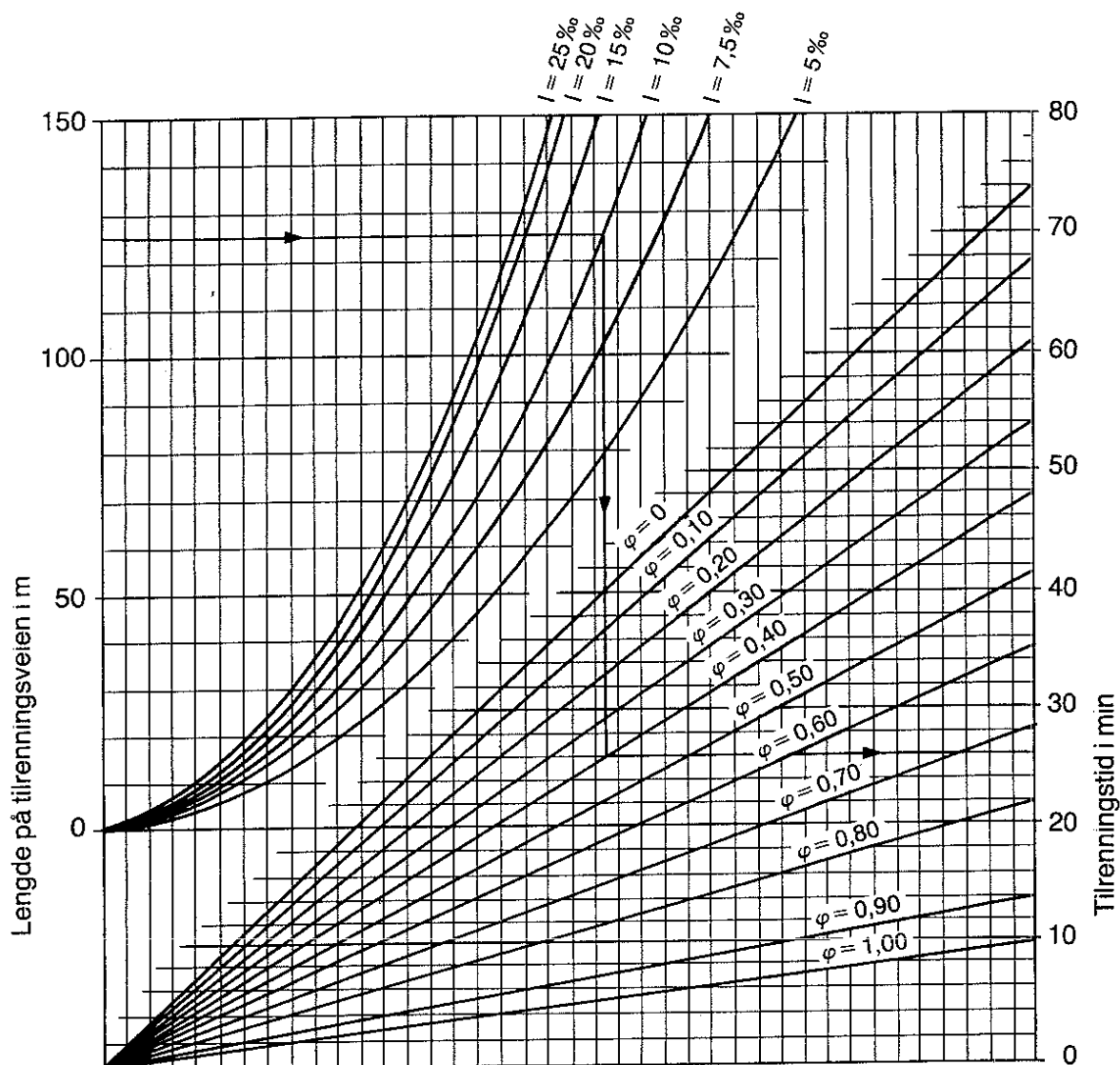
Figur 8. Beregning av tilrenningstid for avrenning på overflaten (SFT TA-550)
